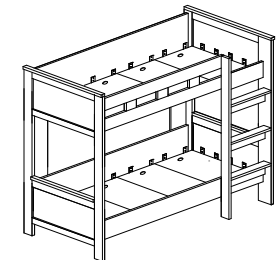
ELINE MODEL : BED 71-S5V ITEM : BUNKER BED L 208 X D 112.5 X H 175cm
