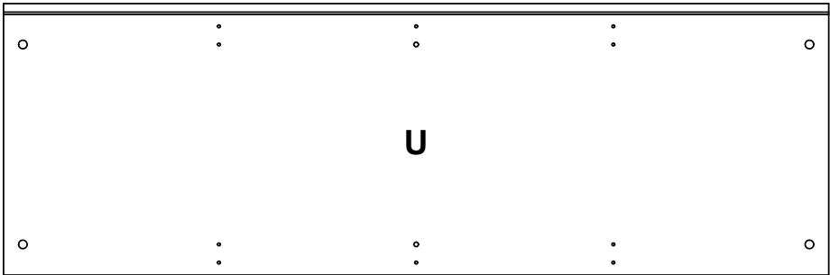
1452x478x18mm
