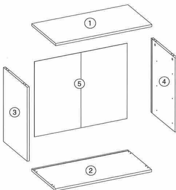
Dimensions / Abmessung in mm/
